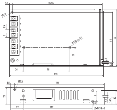
Рис 4. Габаритные размеры (MPS-150W-12)
