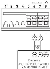
Рис. 15 — Подключение для измерения по току THT-103
