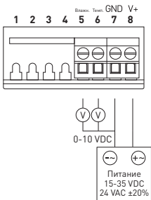
Рис. 14 — Подключение для измерения по напряжению THT-103
