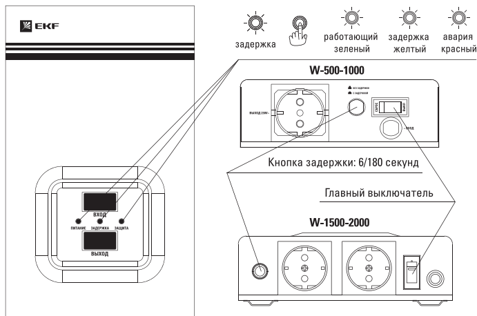
Рис. 2 Внешний вид стабилизатора W-500-2000
